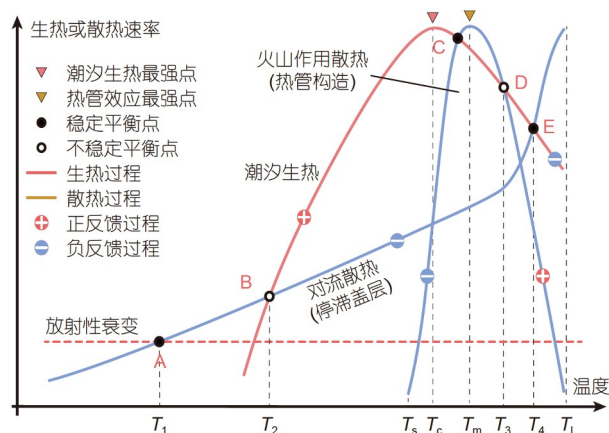
图4 木卫一热收支之间与内部温度之间的反馈关系示意图。 T_s 、 T_1 、 T_c 和 T_m 分别为地幔固相线温度、液相线温度以及潮汐作用和岩浆分离迁移最显著的地幔温度, T_1 、 T_2 、 T_3 和 T_4 分别为木卫一达到生热-散热平衡点时的地幔温度。据文献 [81,82] 修改和补充
